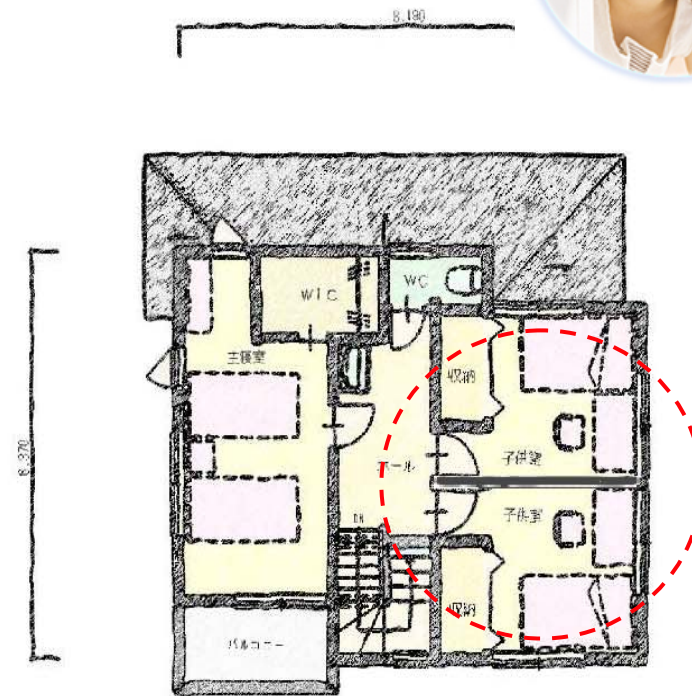
2階平面図
